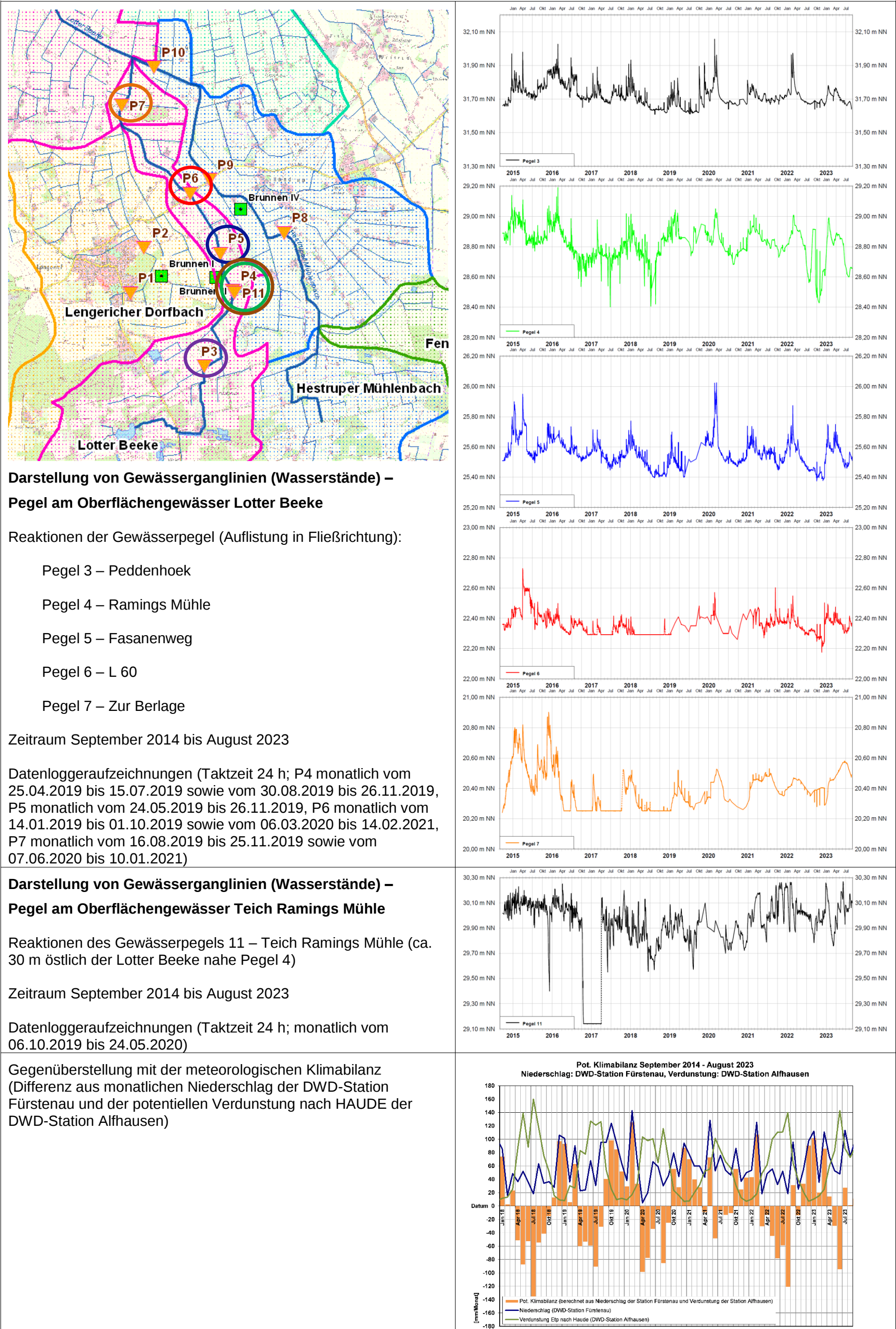
Anlage 3.2.1 – Darstellung von Gewässerganglinien (Wasserstände) ab September 2014 – Pegel Lotter Beeke und Mühltich – Gegenüberstellung der monatlichen meteorologischen Klimabilanz und den Monatsniederschlägen
