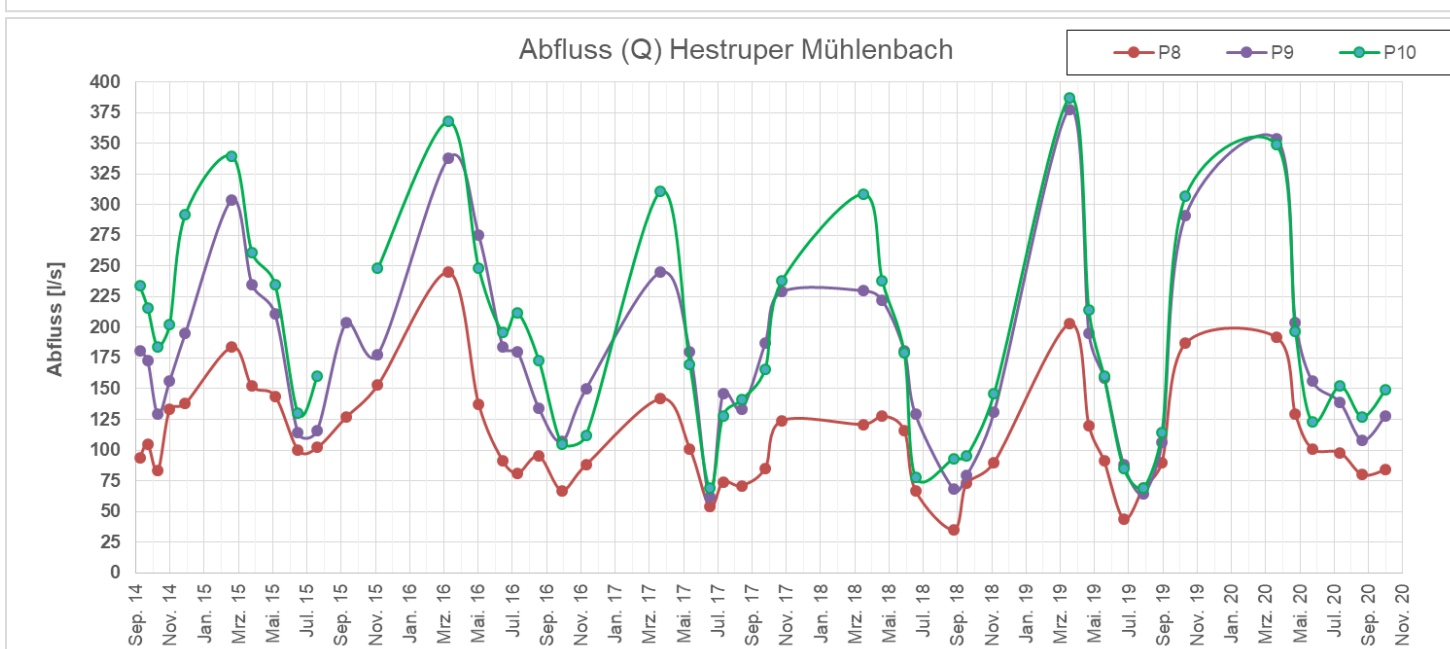
Wasserstände und Abflussmengen am Hestruper Mühlenbach
